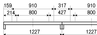
直付連結使用例
