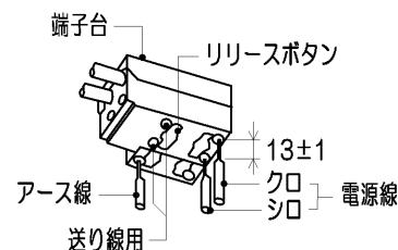
(適合電線φ1.6, φ2.0 単線) 第3図
