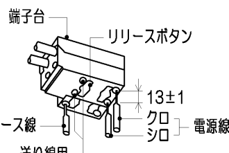
第4図 (適合電線φ1.6, φ2.0 単線)
