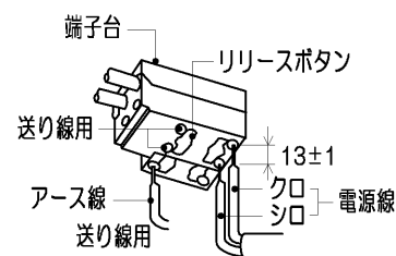
第1図 (適合電線φ1.6, φ2.0 単線)
