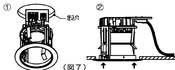
取付け金具の固定方法
