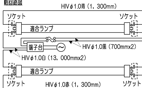
略回路図
