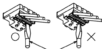
第8図 マイナスイドライバー
