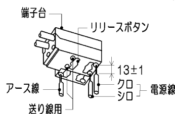
第4図 (適合電線φ1.6, φ2.0 単線)
