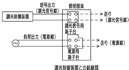
調光制御装置との結線図
