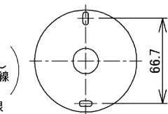
図-3サポート取付ピッチ
