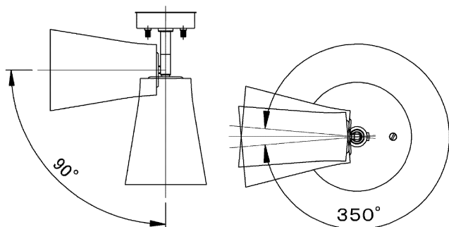
図-4 セード可動範囲
