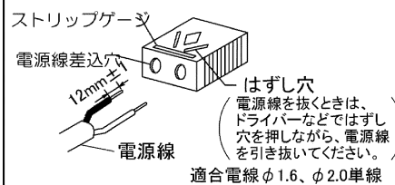
図-2 SL端子台
