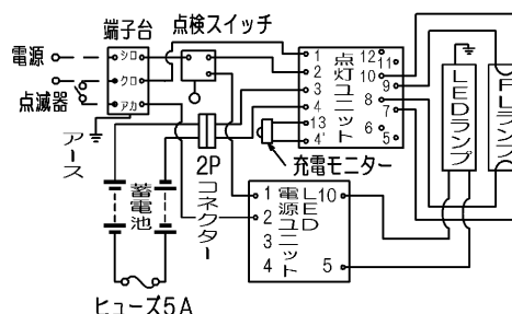
結線図：LEDTS-21830L-LJ1
