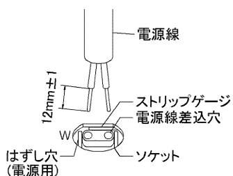
適合電線 \phi 1.6 、 \phi 2.0 Cu単線 図-2 電源線接続方法
