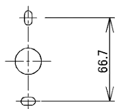
図-3 取り付け寸法図
