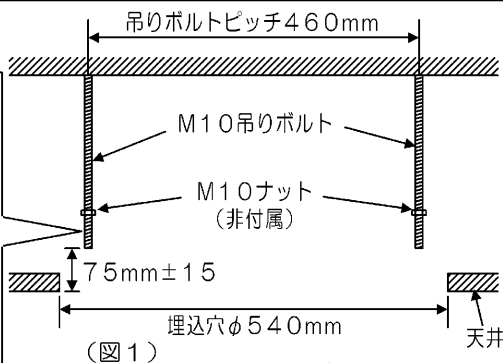
取付け金具の固定方法
