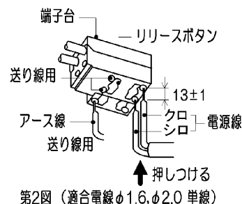
第2図 (適合電線φ1.6, φ2.0 単線)
