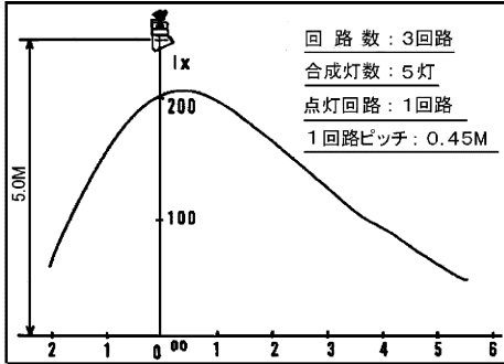
ボーダーライト 形名：AL-BLQ-212-3C
