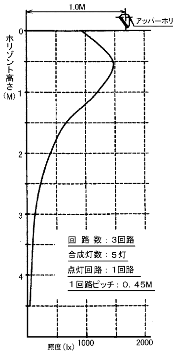
アッパーホリゾンライト 形名：AL-UHQ-212-3C
