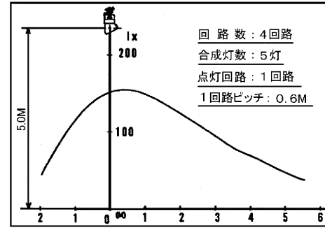
ボーダーライト 形名：AL-BLQ-212-4C
