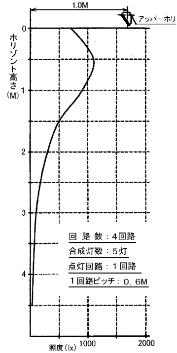
アッパーホリゾンライト 形名：AL-UHQ-212-4C
