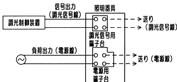
調光制御装置との結線図
