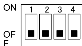
DF-70162-PD コントルクス設定スイッチ図
