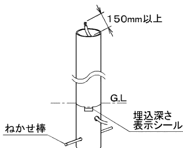
図-2 ポールの埋込み
