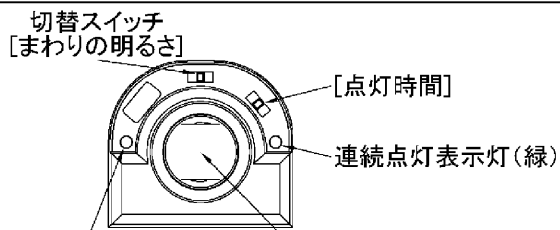
照度センサー 人感センサー検知部(レンズ)
