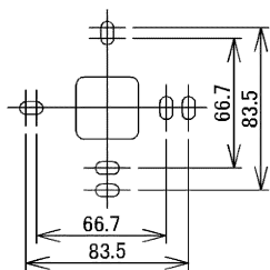
図-3 取り付け寸法図
