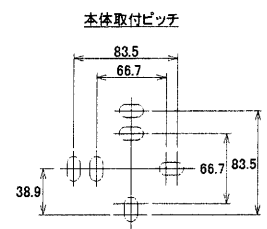
(図2) 保護チューブの取付方
