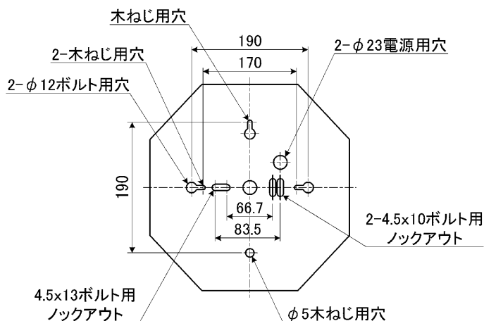
背面仕様図
