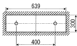
FRS-22751M 単体取付
