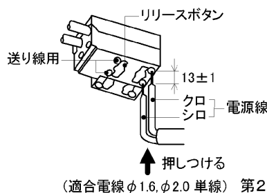
(適合電線φ1.6, φ2.0 単線) 第2図
