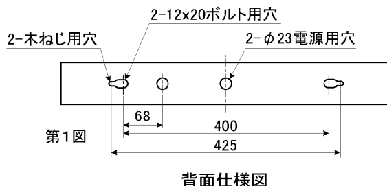
背面仕様図
