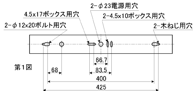
背面仕様図
