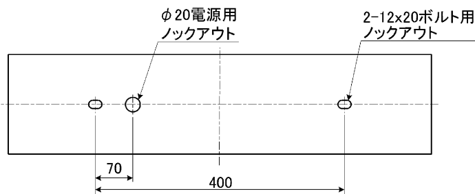
背面仕様図
