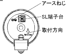
図-2 フランジ内面
