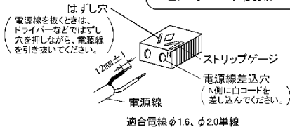
図-1 SL端子台
