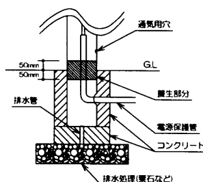
コンクリート施工の場合
