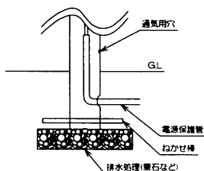
ねかせ棒仕様の施工の場合
