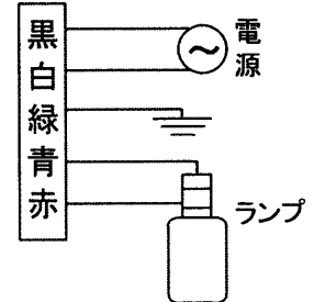
結線図
