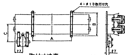
取付寸法表
