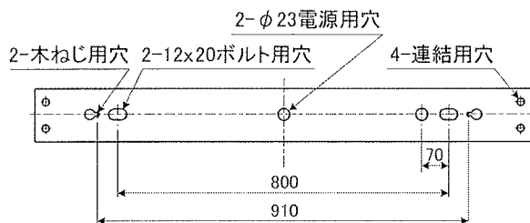
背面仕様図
