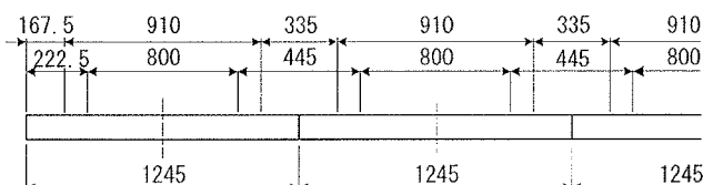
連結寸法図
