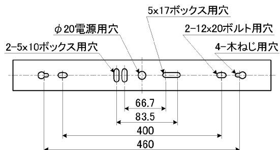
背面仕様図
