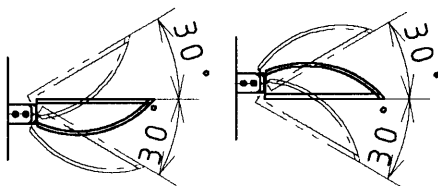
角度可変アーム壁付の場合
