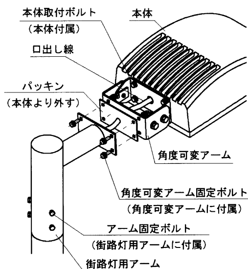
街路灯角度可変アーム付
