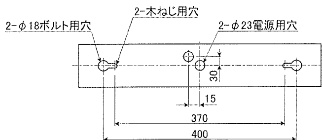
背面仕様図
