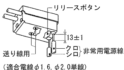
非常用電源端子台
