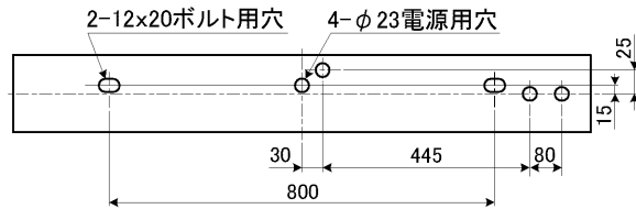
背面仕様図
