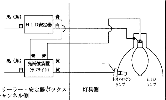
Ⓑ始動時、再始動時及び常夜灯としてもネオハロゲンランプを点灯する場合の結線図
