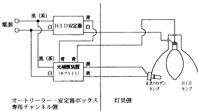
Ⓐ始動時、再始動時のみネオハロゲンランプを点灯する場合の結線図
