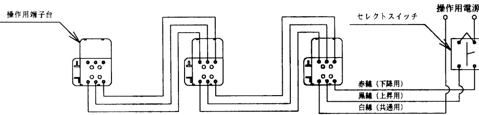
Ⓐ始動時、再始動時のみネオハロゲンランプを点灯する場合の結線図
