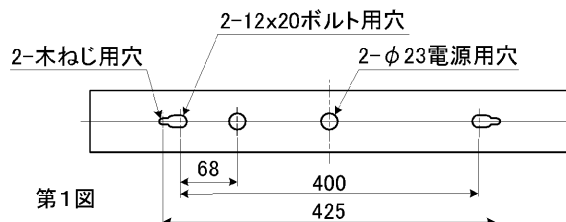
背面仕様図
