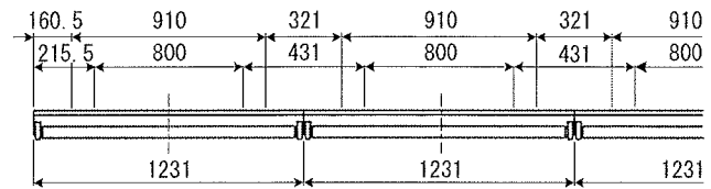
連結寸法図
