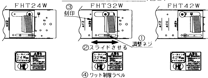
各ランプ別ソケット台位置(図2)
