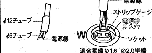
図-1 電源線接続方法
