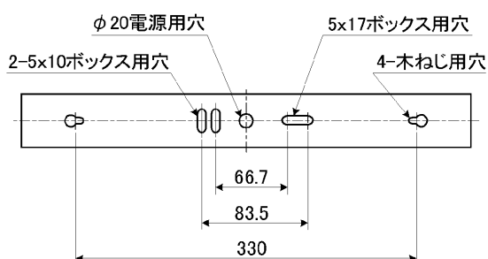
背面仕様図
