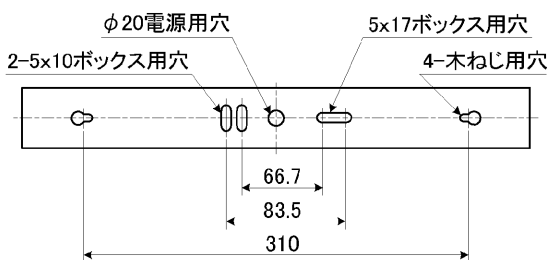
背面仕様図
