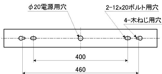
背面仕様図
