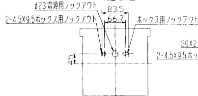
(図4)(単位:mm)
