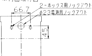
(図2)(単位:mm)
