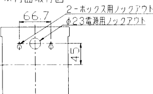
(図2)(単位:mm)
