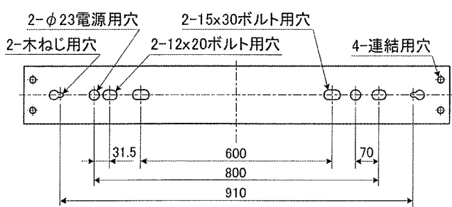
FHT-91311M-PR9 背面仕様図
