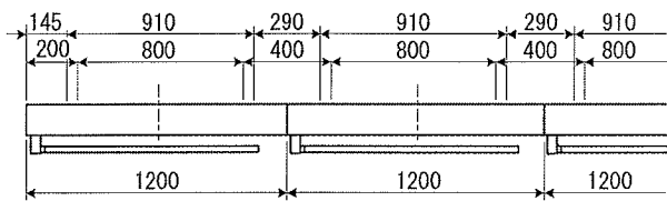
FHT-91311M-PR9 連結寸法図
