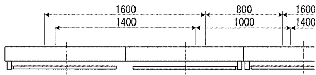
FHT-92311M-PR9 連結寸法図
