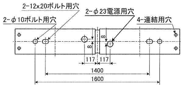
FHT-92311M-PR9 背面仕様図
