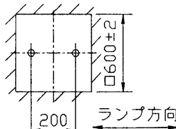
FHR-54320-PN9 器具取付ボルトの寸法 器具内寸法 (A寸法) 40mm
