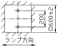
FHR-53320-PN9 器具取付ボルトの寸法 器具内寸法 (A寸法) 30mm
