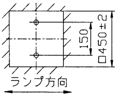
FHR-33320-PR9 器具取付ボルトの寸法 器具内寸法 (A寸法) 30mm
