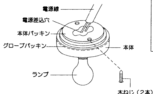
(図1) 電源線接続方法
