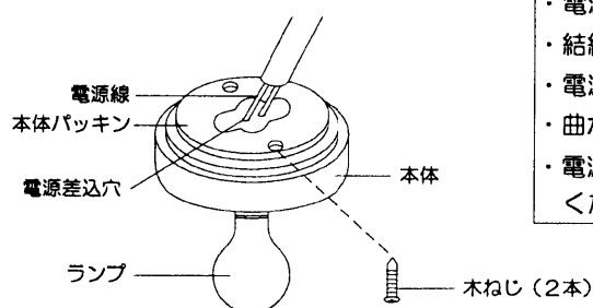
(図1) 電源線接続方法
