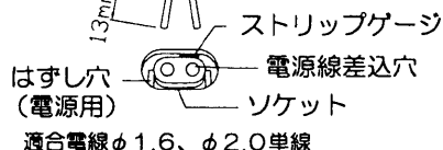
(図1) 電源線接続方法
