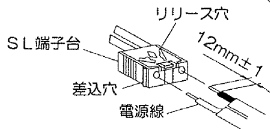
適合電線φ1.6、φ2.0単線 (図3) 電源線接続方法
