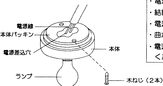
(図1) 電源線接続方法
