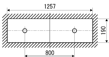
単体取付
