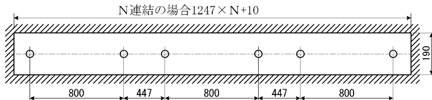
連結取付
