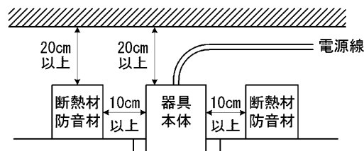
連結取付
